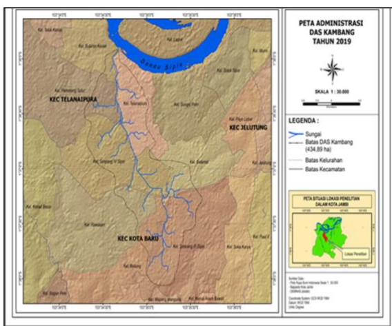
Gambar 1. Daerah Aliran Sungai Kambang
