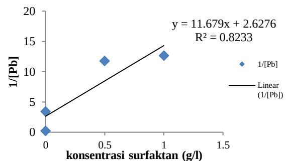
Gambar 4. Grafik 1/[Pb] terhadap konsentrasi (kinetika reaksi) untuk Soil Washing
