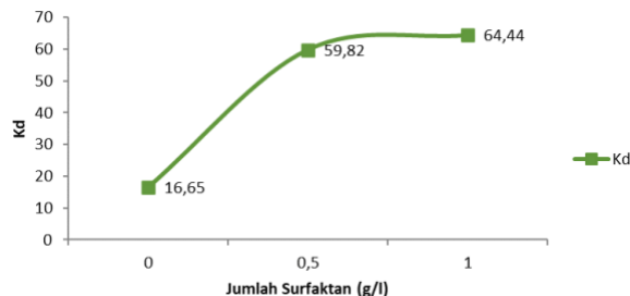
Gambar 5. Grafik Perubahan Nilai Koefisien Distribusi (KD) Logam Pb terhadap Variasi Konsentrasi Surfaktan pada Tanah Loamy Sand
