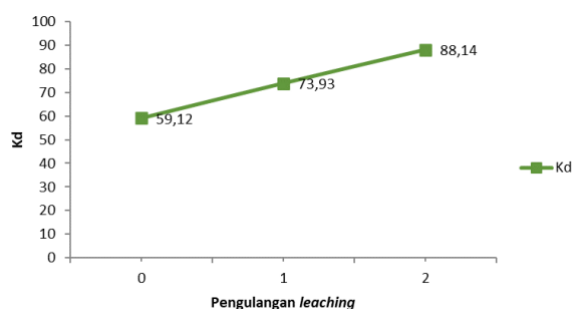
Gambar 6. Grafik Perubahan Nilai Koefisien Distribusi (Kd) Logam Timbal (Pb) terhadap Variasi Pengulangan leaching pada Tanah Loamy Sand
