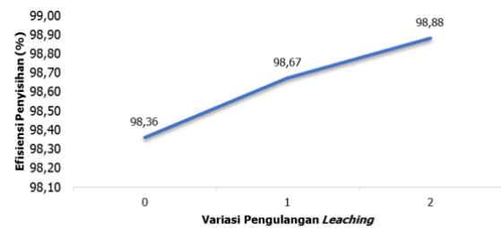
Gambar 3. Grafik Pengaruh Variasi pengulangan soil washing terhadap Penyisihan Timbal (Pb) pada Tanah Loamy Sand
