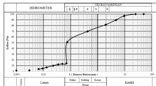
Gambar 2. Grafik Distribusi Ukuran Tanah
