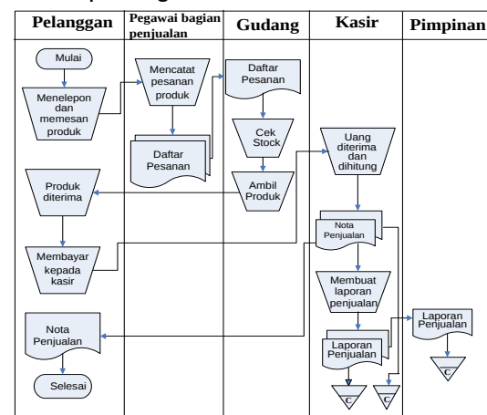
Gambar 2 Flowchart Dokumen Sistem
